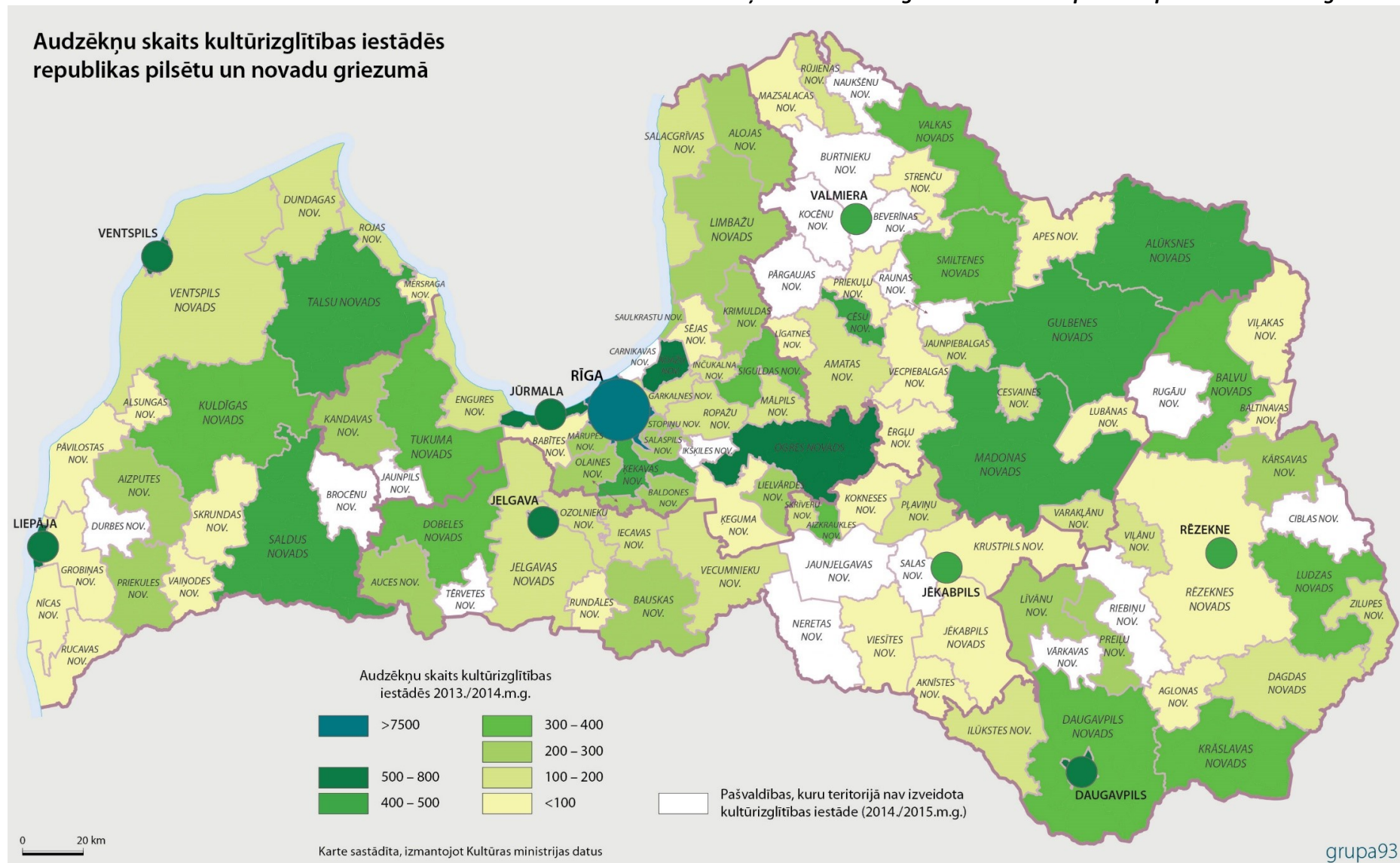
12.att. Audzēkņu skaits kultūrizglītības iestādēs republikas pilsētu un novadu griezumā
